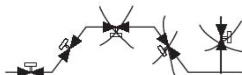
Схема расположения клапанов ДУ65-200 на трубопроводе.
