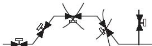
Схема расположения клапанов ДУ15-50 на трубопроводе.
