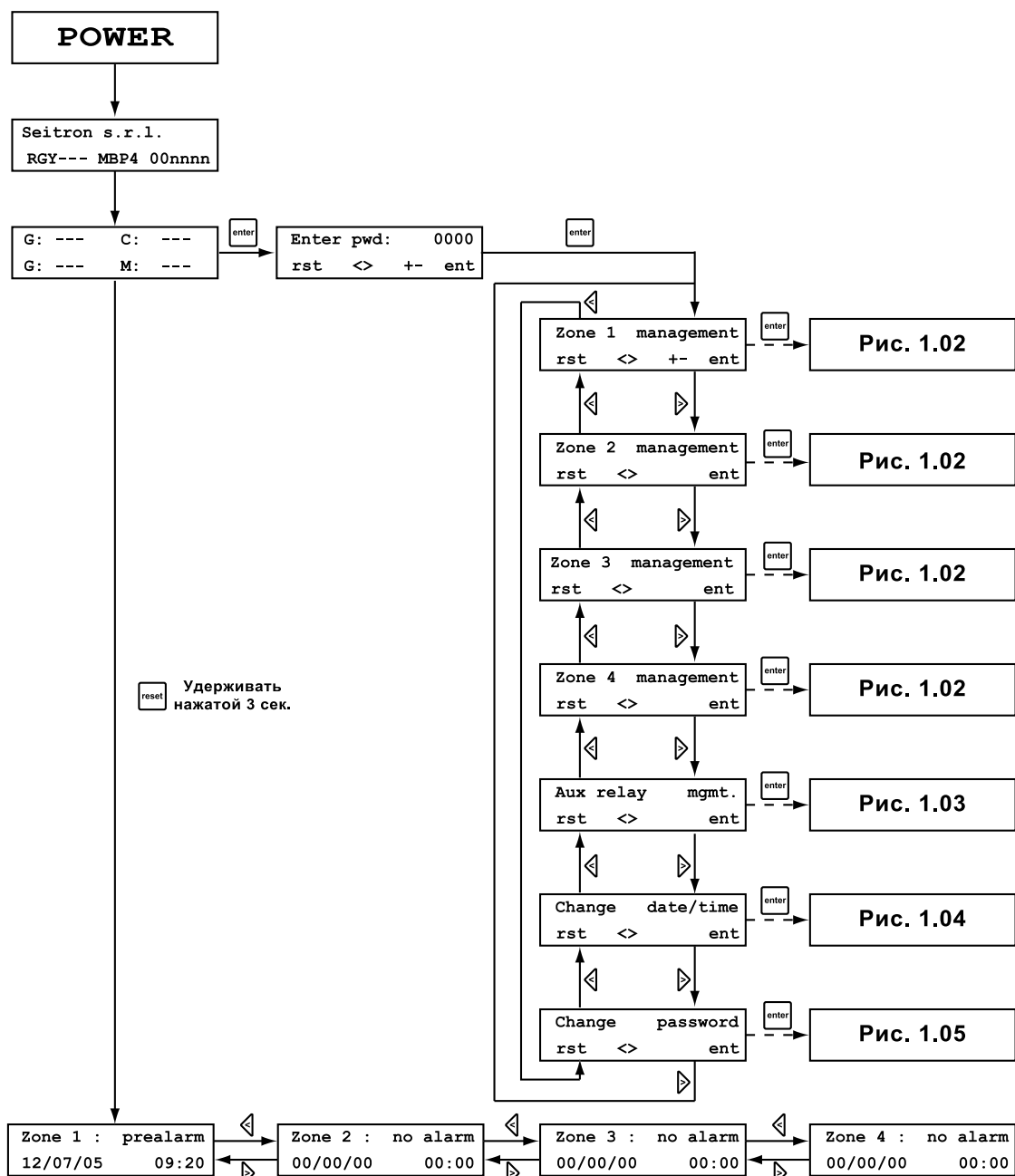
РИС. 1.01 КОНФИГУРАЦИЯ ПАРАМЕТРОВ
